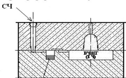
Обробка розплаву в реакційній камері з модифікатором у піщаній формі
