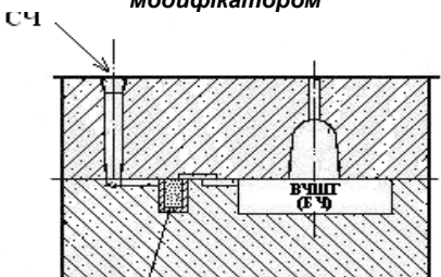
Обробка розплаву в реакційній камері, виконаній у вигляді пінополістиролової оболонки з модифікатором
