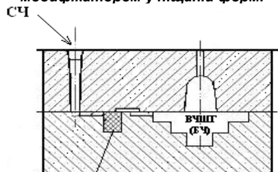
Обробка розплаву в реакційній камері, виконаній у вигляді пінополістиролового патрону з модифікатором
