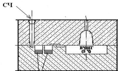
Подвійна обробка розплаву в реакційній камері з модифікатором у піщаній формі
