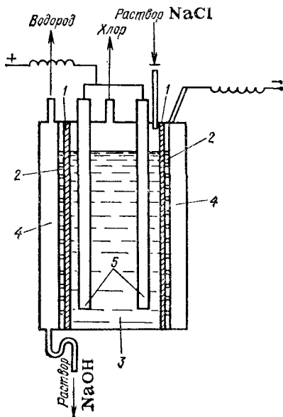
Рис. 154. Схема электролизера с вертикальной диафрагмой:
