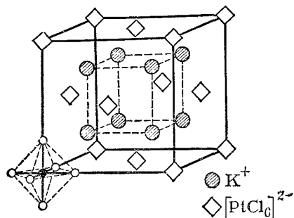
Рис. 159. Кристаллическая решетка K_2[PtCl_6] .
