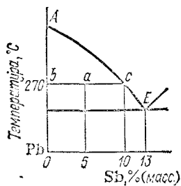
Рис. 149. Часть диаграммы состояния системы Pb — Sb
