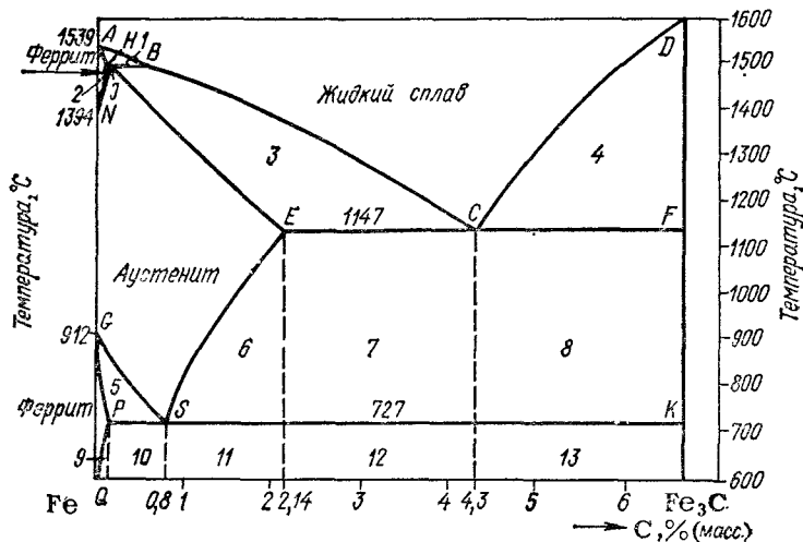
Рис. 168. Диаграмма состояния системы железо — углерод.
