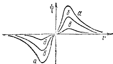
Рис. 15. График волновой функции 2p -электрона.
