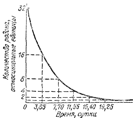
Рис. 25. Зависимость количества нераспавшегося радона от времени.
