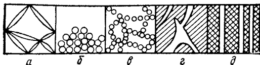
Рис. 89. Связнодисперсные (а — в) и капиллярнодисперсные (г, д) системы:
