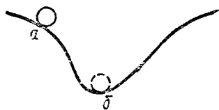
Рис. 69. Шарик самопроизвольно скатывается из положения a в положение б .
