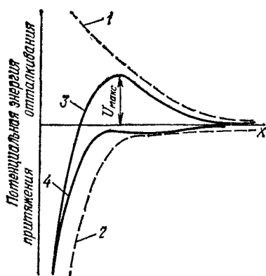
Рис. 103. Потенциальная энергия взаимодействия между двумя одинаково заряженными частицами: 1 — электрическое отталкивание ( U_э ); 2 — дисперсионное притяжение ( U_д ); 3 — результирующая энергия взаимодействия ( U ); 4 — то же, но при более крутом падении кривой 1; x — расстояние между частицами; U_{\max} — потенциальный барьер взаимодействия дисперсных частиц.
