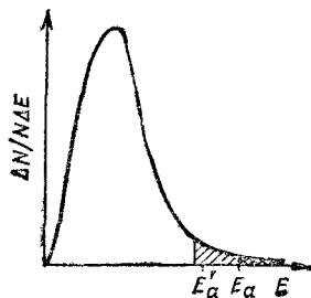
Рис. 67. Влияние катализатора на число активных молекул:
