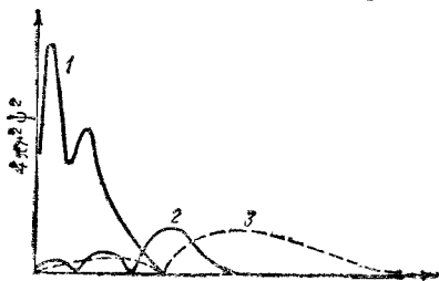
Рис. 21. График радиального распределения вероятности в атоме натрия.
