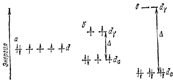
Рис. 162. Распределение электронов иона \text{Co}^{3+} по d -орбиталям:
