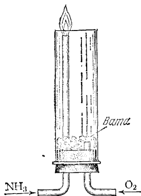
Рис. 114. Прибор для демонстрации горения аммиака в кислороде.
