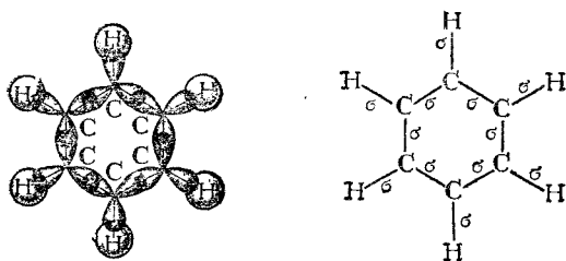
Рис. 131. Схема образования \sigma -связей в молекуле бензола.
