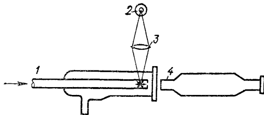
Рис. 92. Схема поточного ультрамикроскопа Б. В. Дерягина и Г. Я. Власенко:
