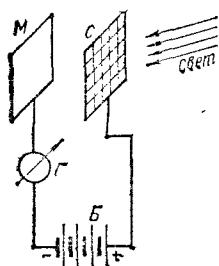
Рис. 4. Схема установки для наблюдения фотоэлектрического эффекта:
