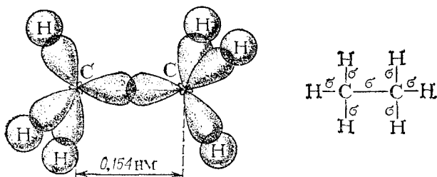
Рис. 124. Схема образования \sigma -связей в молекуле этана.
