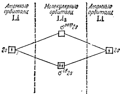
Рис. 49. Энергетическая схема образования молекулы лития Li_2 .
