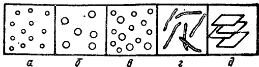
Рис. 88. Свободнодисперсные системы:
