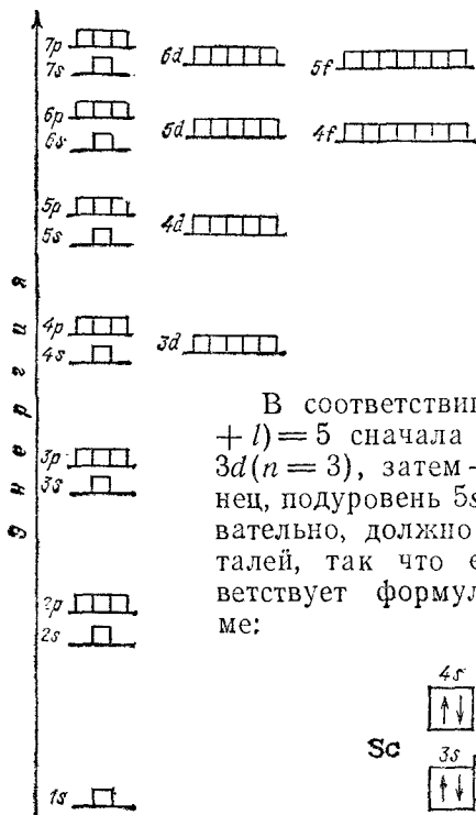
Рис. 22. Последовательность заполнения электронных энергетических подуровней в атоме.
