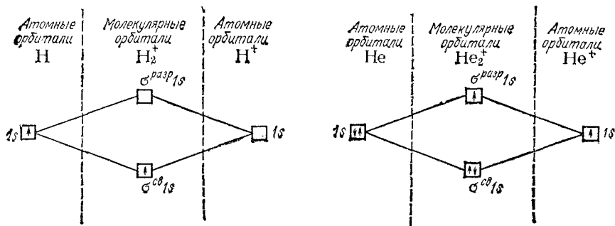
Рис. 47. Энергетическая схема образования молекулярного иона водорода \text{H}_2^+ .
