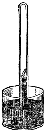
Рис. 119. Прибор для демонстрации поглощения аммиака углем.
