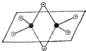
Рис. 165. Схема пространственного строения молекулы Al_2Cl_6 :
