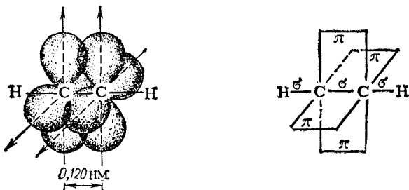
Рис. 127. Схема образования \pi -связей в молекуле ацетилена.
