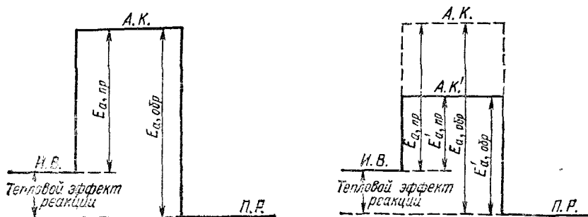
Рис. 65. Энергетическая схема реакции:
