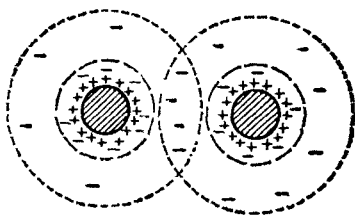
Рис. 102. Схема перекрывания ионных атмосфер двух коллоидных частиц.
