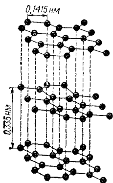
Рис. 118. Структура графита.
