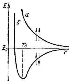
Рис. 26. Энергия системы, состоящей из двух атомов водорода: a — при одинаково направленных спинах электронов; б — при противоположно направленных спинах; E_0 — энергия системы из двух невзаимодействующих атомов водорода; r_0 — межъядерное расстояние в молекуле водорода.
