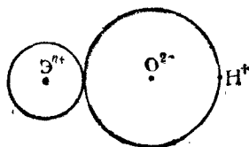
Рис. 108. Ионная схема фрагмента молекулы гидроксида \text{Э}(\text{OH})_n .
