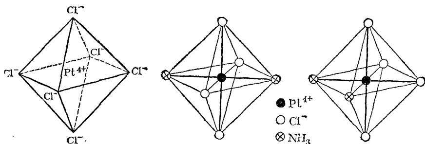
Рис. 157. Пространственное строение комплексного иона [PtCl_6]^{2-} .
