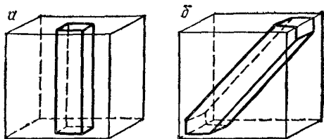
Рис. 60. Бруски, вырезанные из кристаллов каменной соли:
