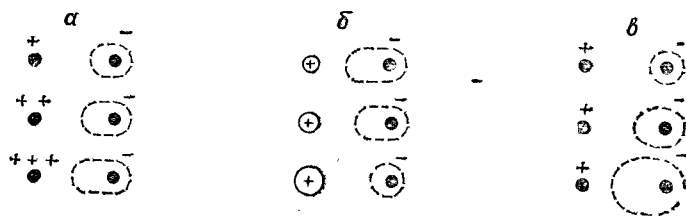
Рис. 55. Схема влияния на поляризацию отрицательных ионов:
