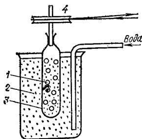
Рис. 91. Схема диализа:
