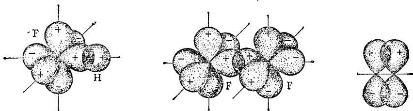
Рис. 32. Схема перекрывания 2p -электронного облака атома фтора и 1s -электронного облака атома водорода при образовании \sigma -связи в молекуле HF: + и - знаки волновой функции.
