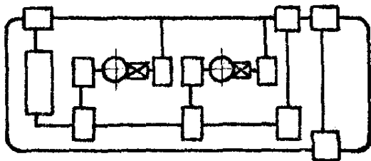
Автоматична лінія для виготовлення форм струшуванням і допресовуванням мод. 4Л22821
