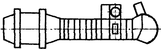
Автоматична піскодувно-пресова лінія вертикального безококового формування мод. АЛ28413
